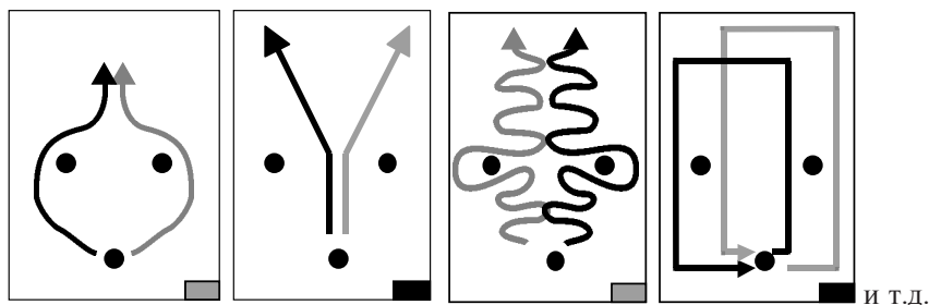
Рис. 20. Тропинки
